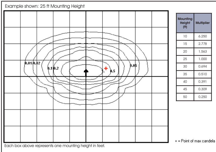
Iso-Illuminance Chart (fc)
